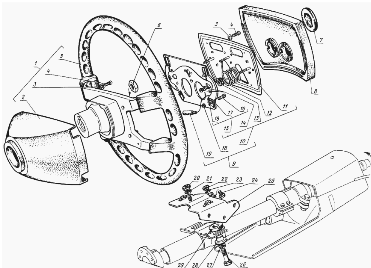
Рис. 43. Колесо рулевого управления, крепление рулевого управления, выключатель звукового сигнала
