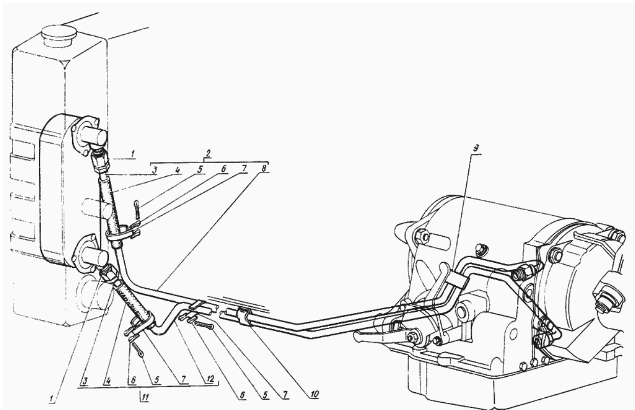
Рис. 29. Система охлаждения коробки передач
