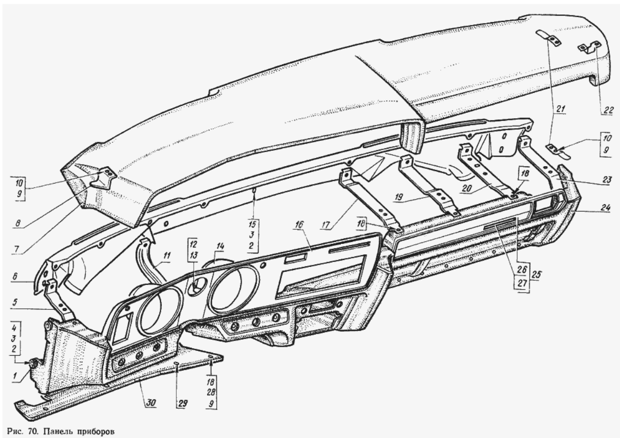
Рис. 70. Панель приборов
