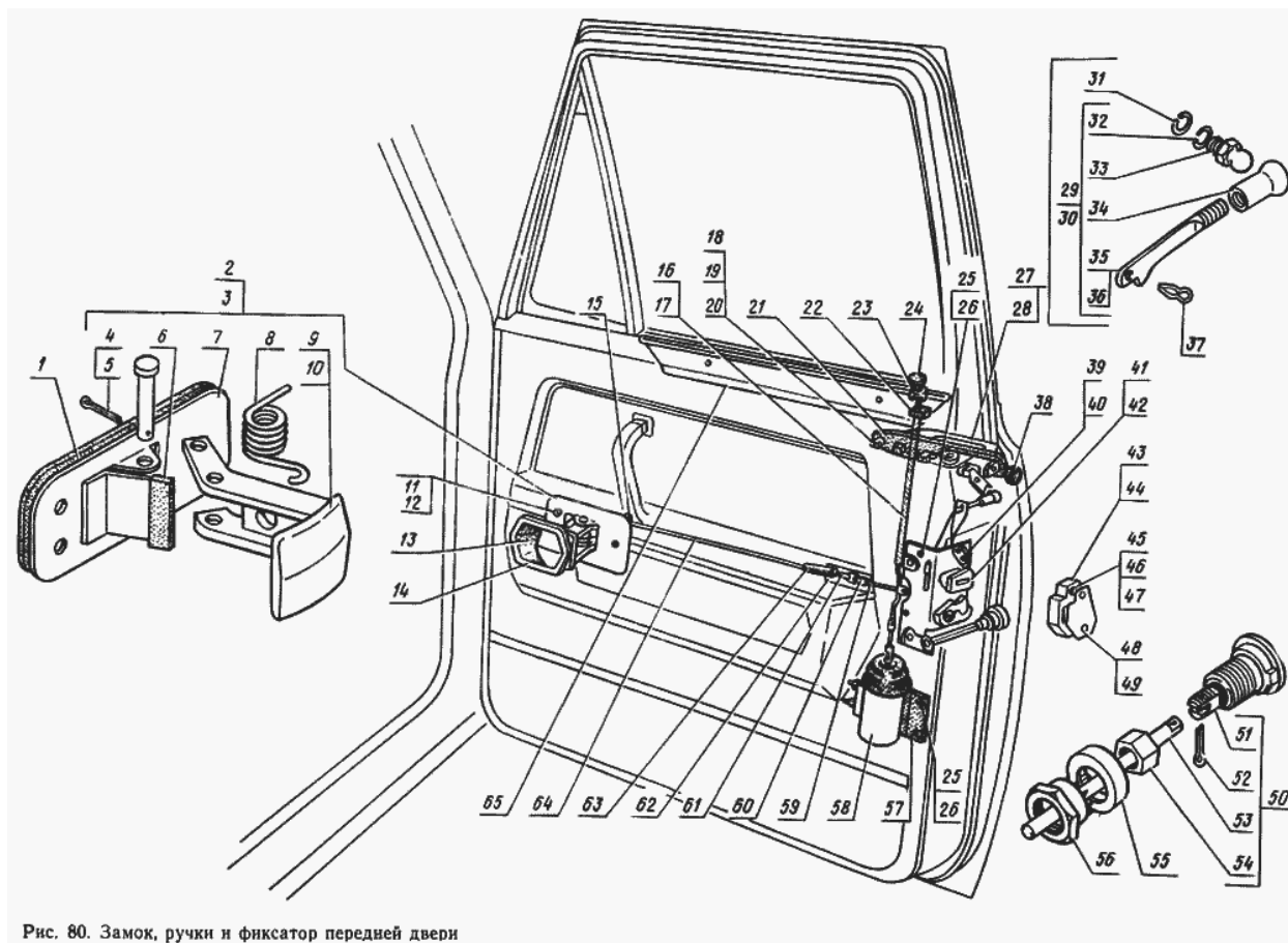
Рис. 80. Замок, ручки и фиксатор передней двери
