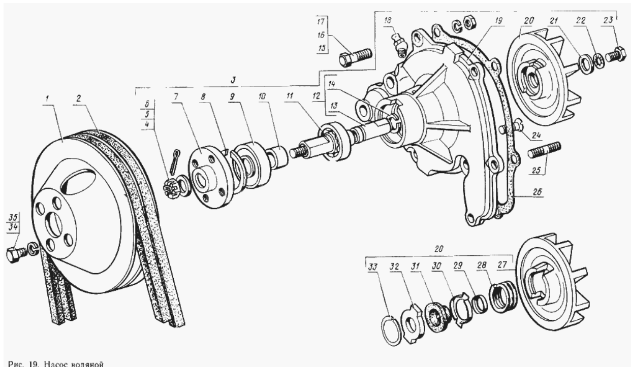
Рис. 19. Насос водяной
