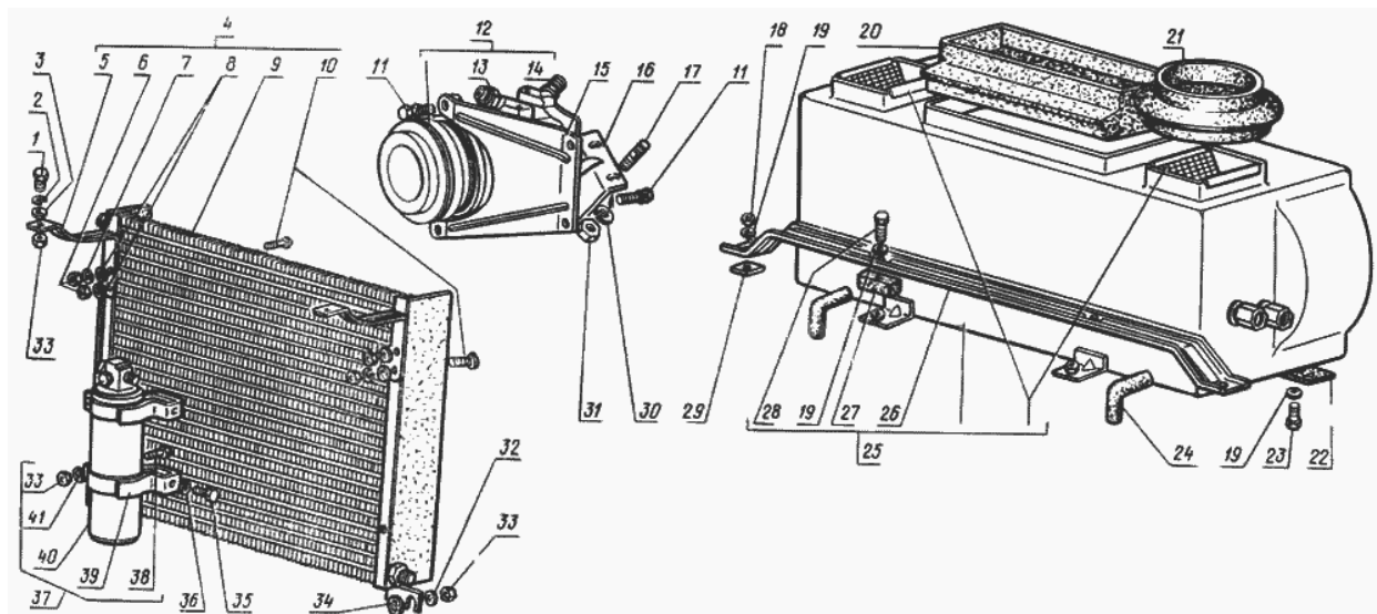
Рис. 94. Компрессор холодильный, конденсатор, ресивер, охладитель воздуха
