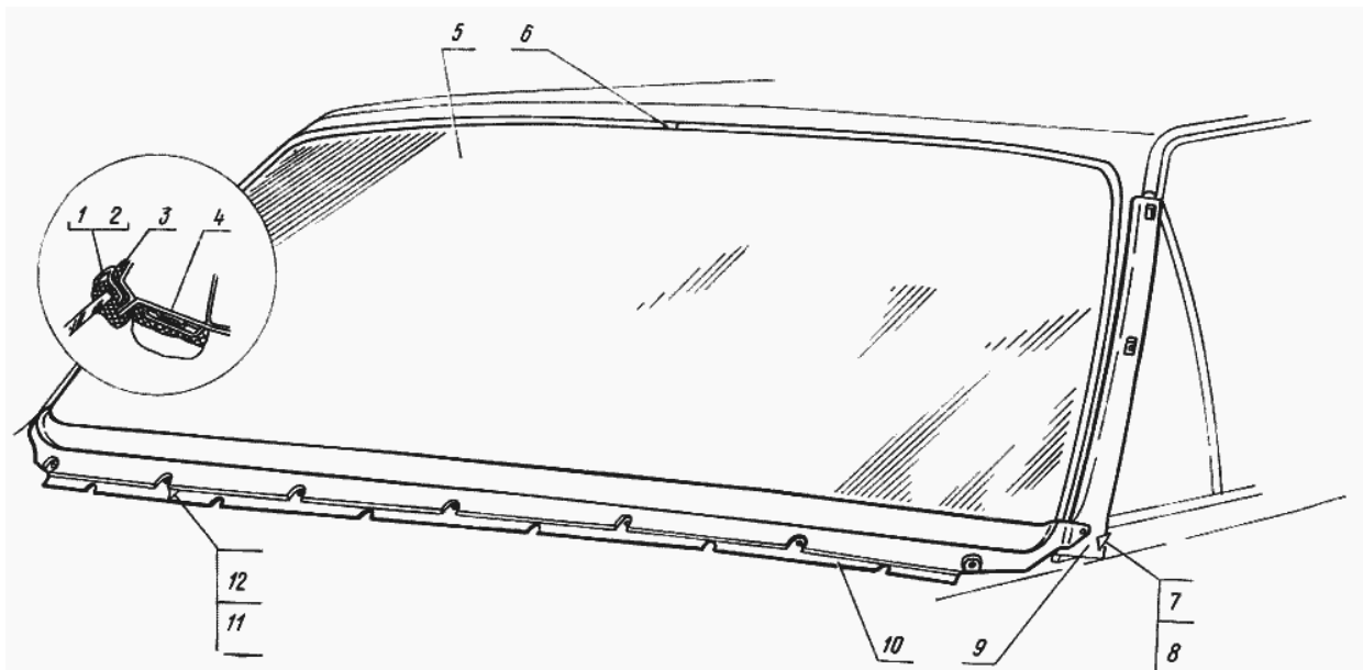
Рис. 68. Стекло и отделочная рамка ветрового окна
