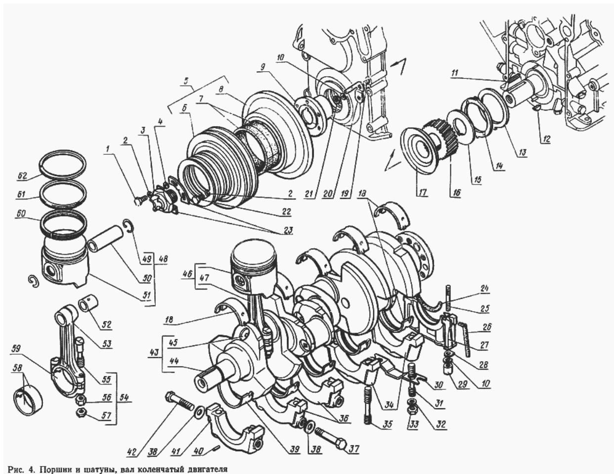
Рис. 4. Поршни и шатуны, вал коленчатый двигателя
