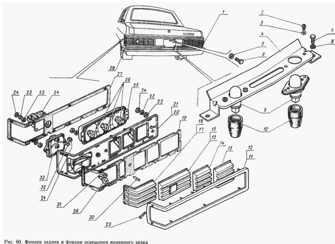
Рис. 60. Фонари задние и фонари освещения номерного знака
