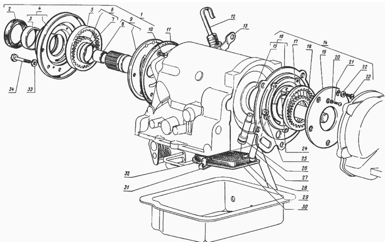
Рис. 22. Насосы масляные автоматической коробки передач
