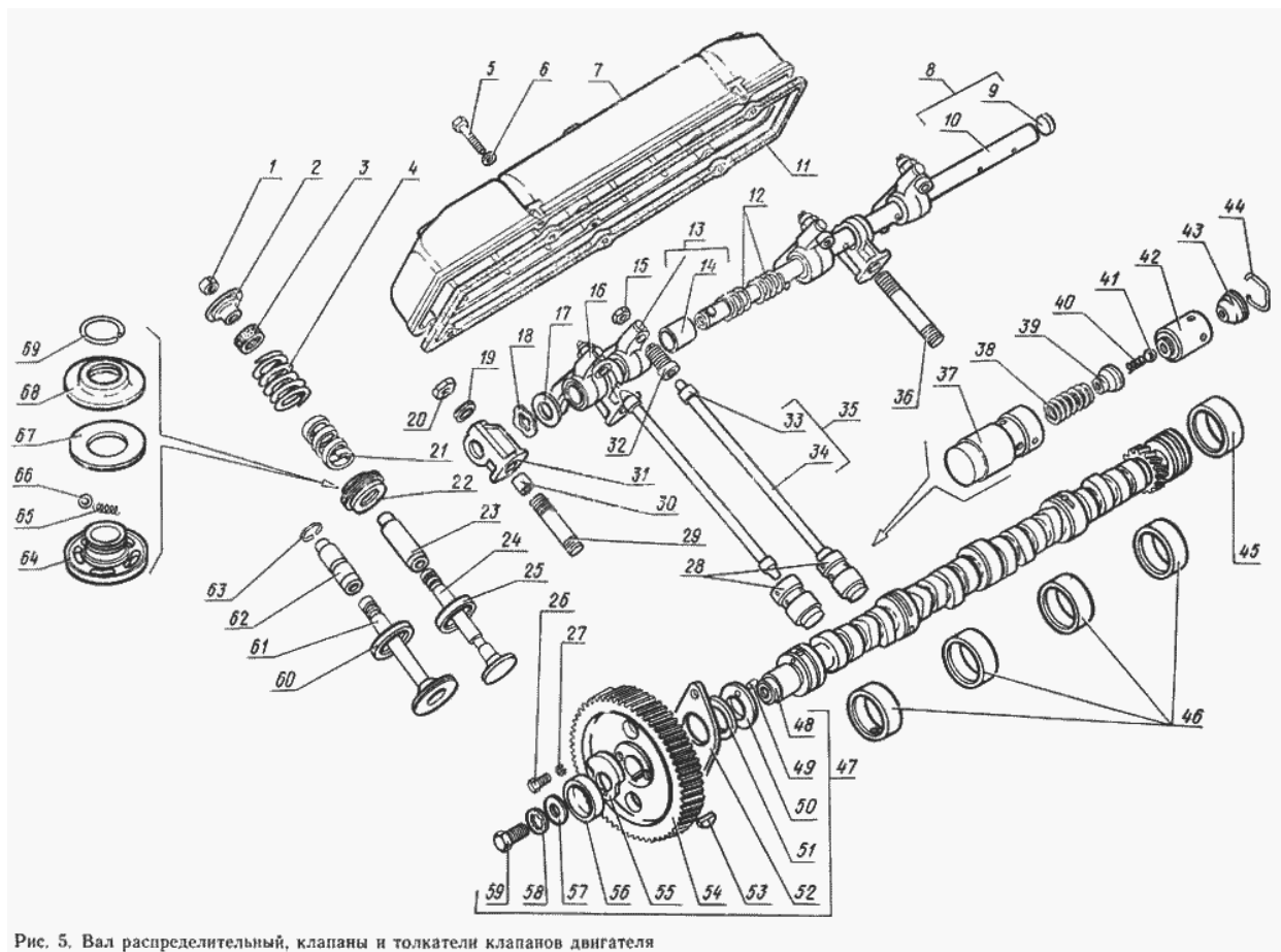
Рис. 5. Вал распределительный, клапаны и толкатели клапанов двигателя
