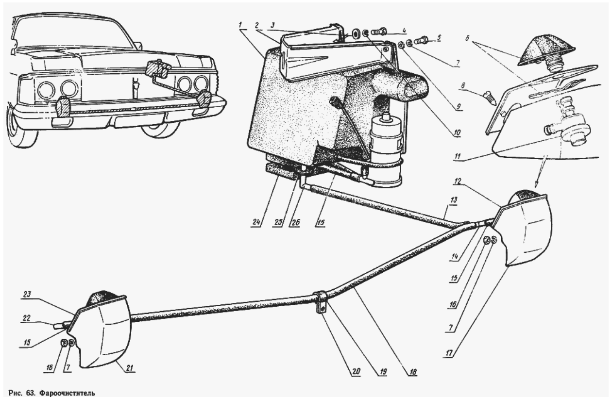
Рис. 63. Фароочиститель
