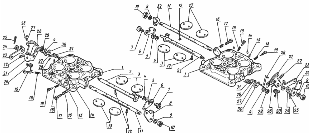
Рис. 14. Карбюратор
