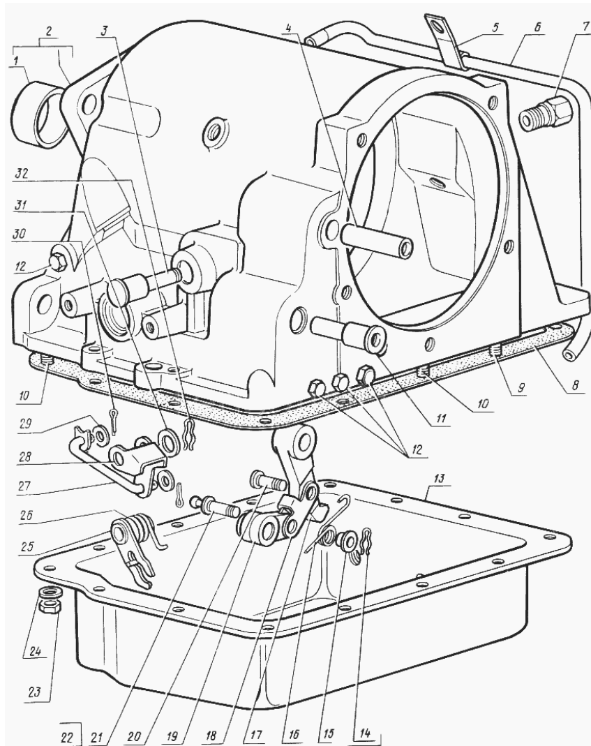
Рис. 24. Картер и поддон автоматической коробки передач
