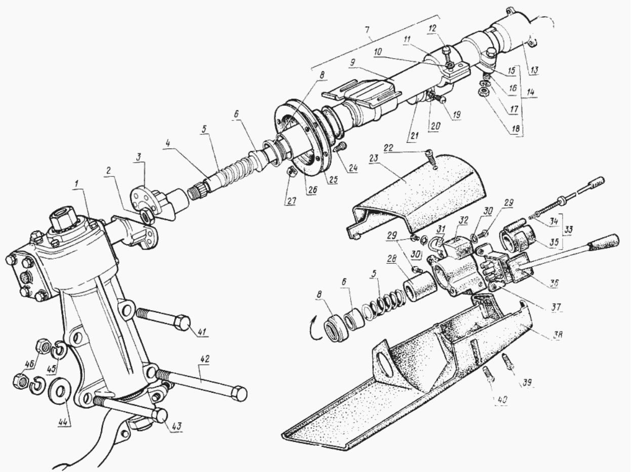
Рис. 42. Управление рулевое
