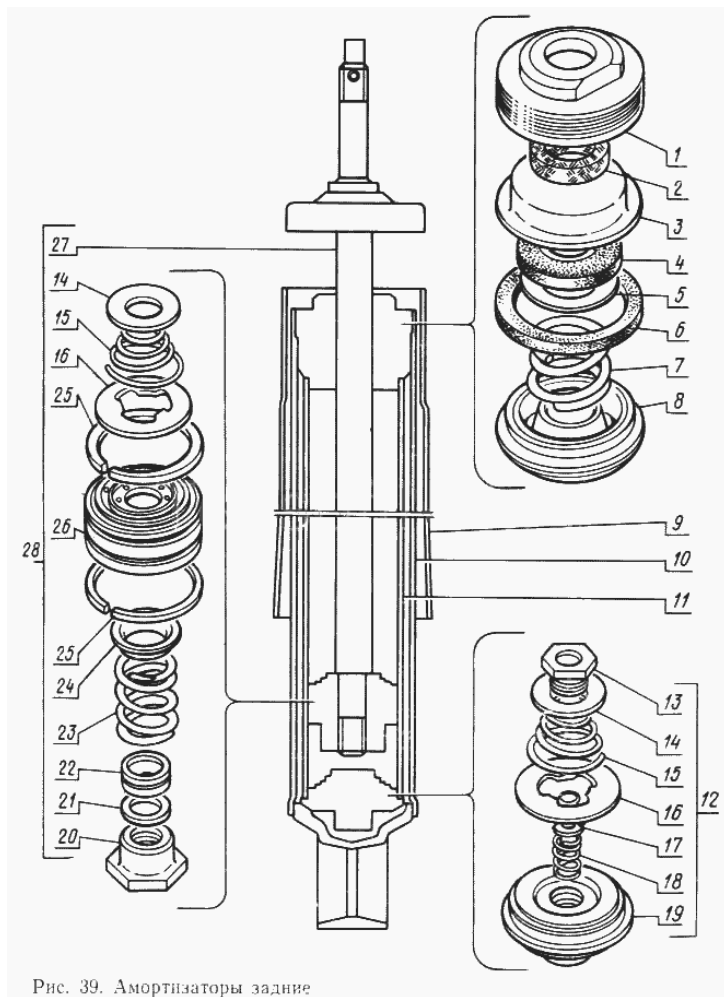
Рис. 39. Амортизаторы задние
