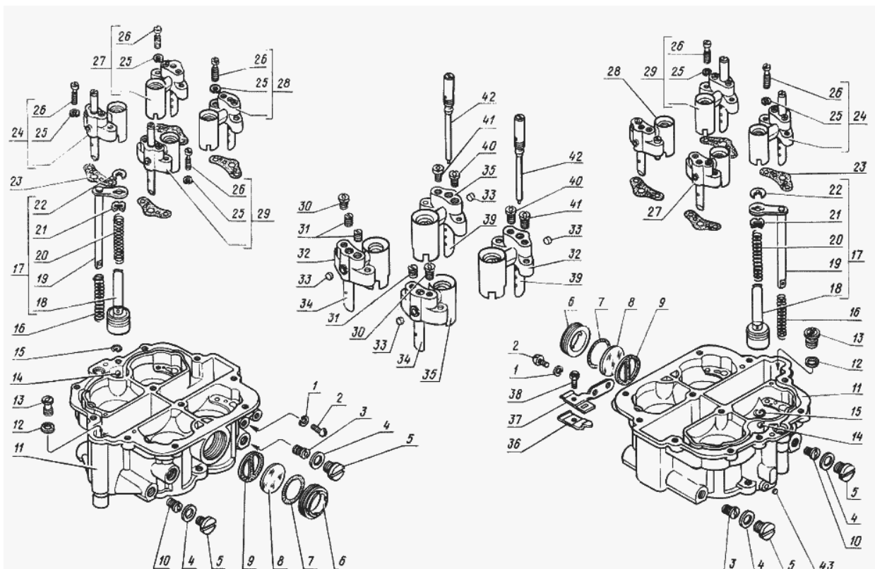
Рис. 13. Карбюратор
