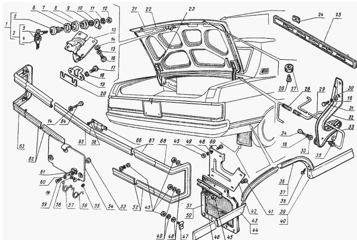
Рис. 74. Задок, крышка багажника, петли крышки багажника, замок багажника, крыло заднее
