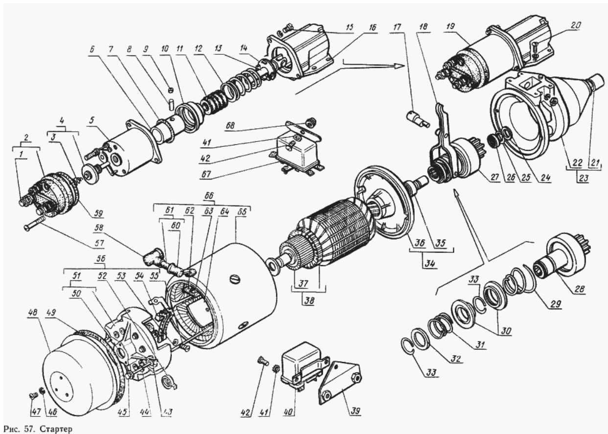
Рис. 57. Стартёр
