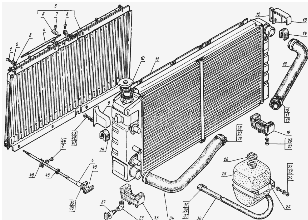
Рис. 18. Радиатор, подвеска радиатора, трубопроводы и шланги, пробка радиатора, краник сливной, жалюзи радиатора и привод и бачок расширительный
