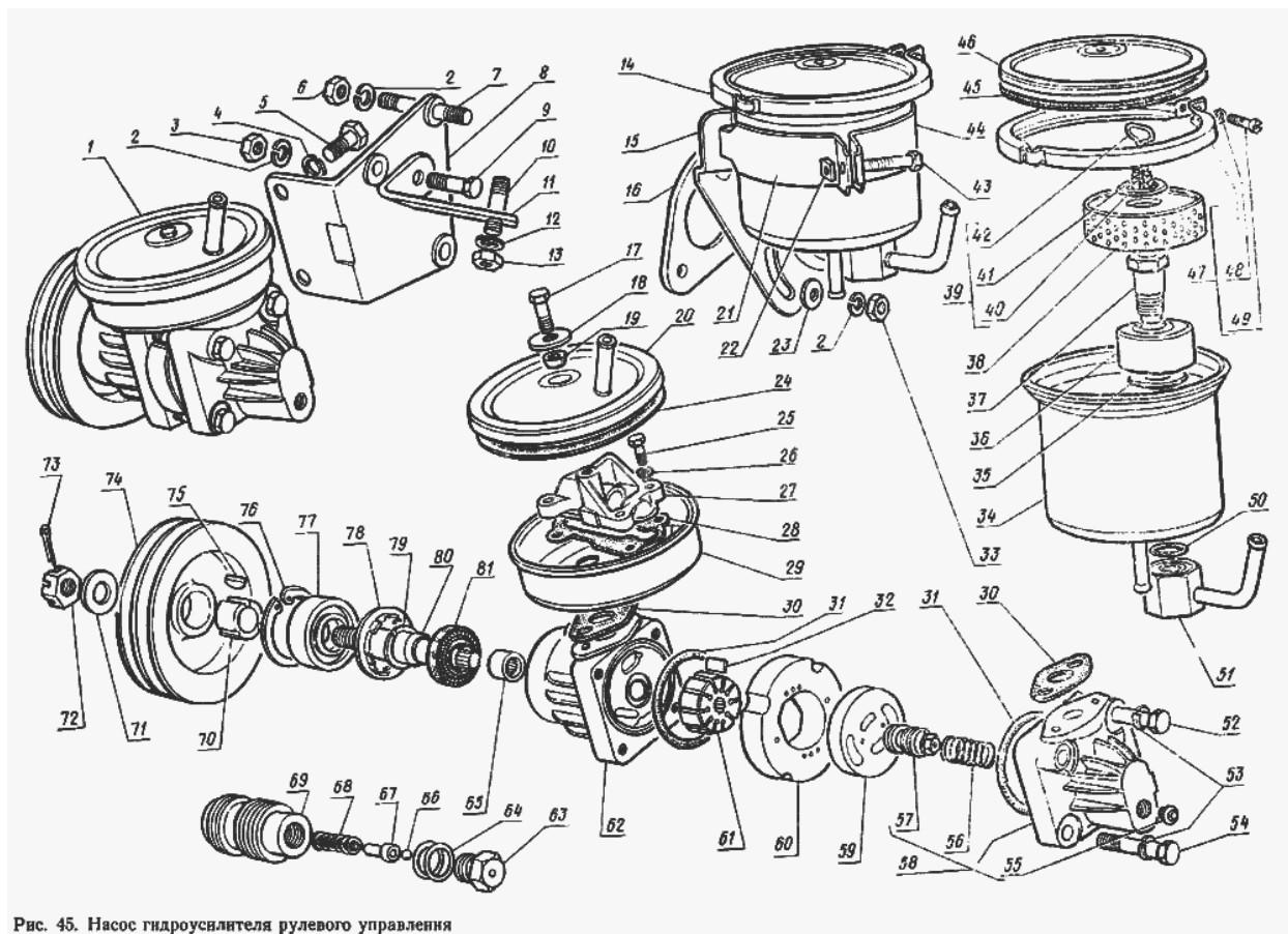
Рис. 45. Насос гидроусилителя рулевого управления
