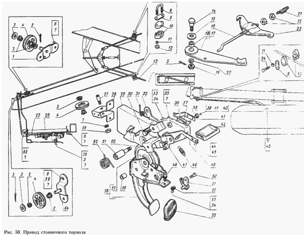
Рис. 50. Привод стояночного тормоза
