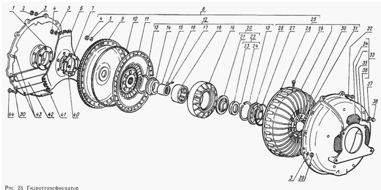
Рис. 23. Гидротрансформатор
