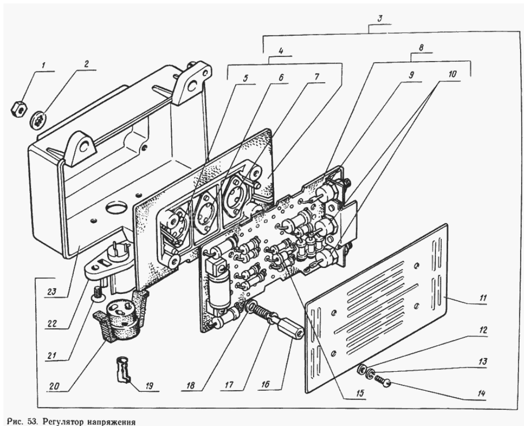
Рис. 53. Регулятор напряжения
