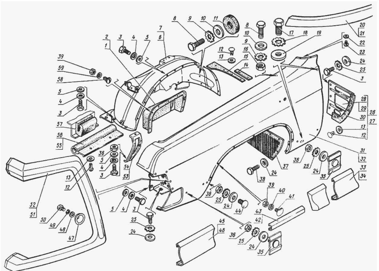
Рис. 99. Крыло переднее
