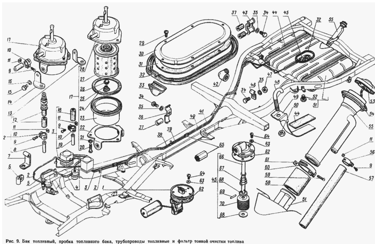
Рис. 9. Бак топливный, пробка топливного бака, трубопроводы топливные и фильтр тонкой очистки топлива
