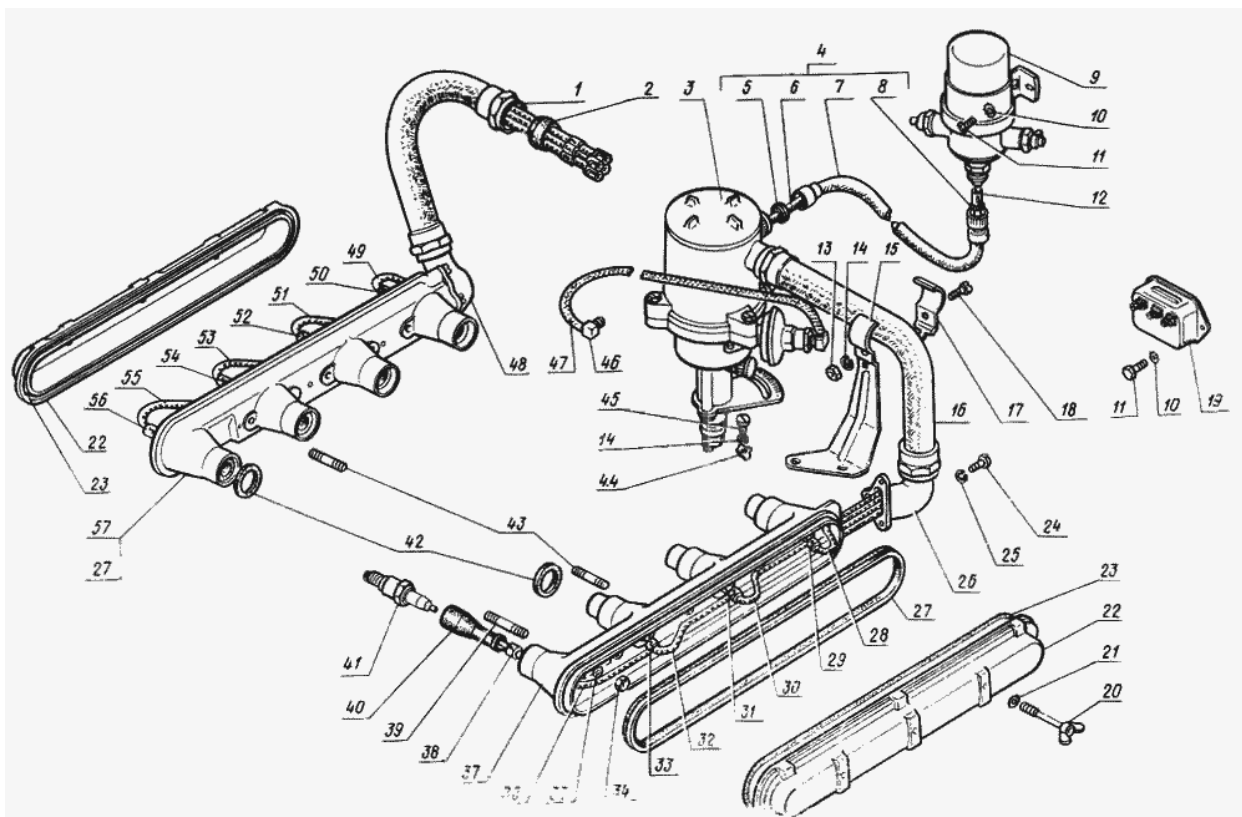
Рис. 55. Катушка, распределитель, свечи и провода зажигания
