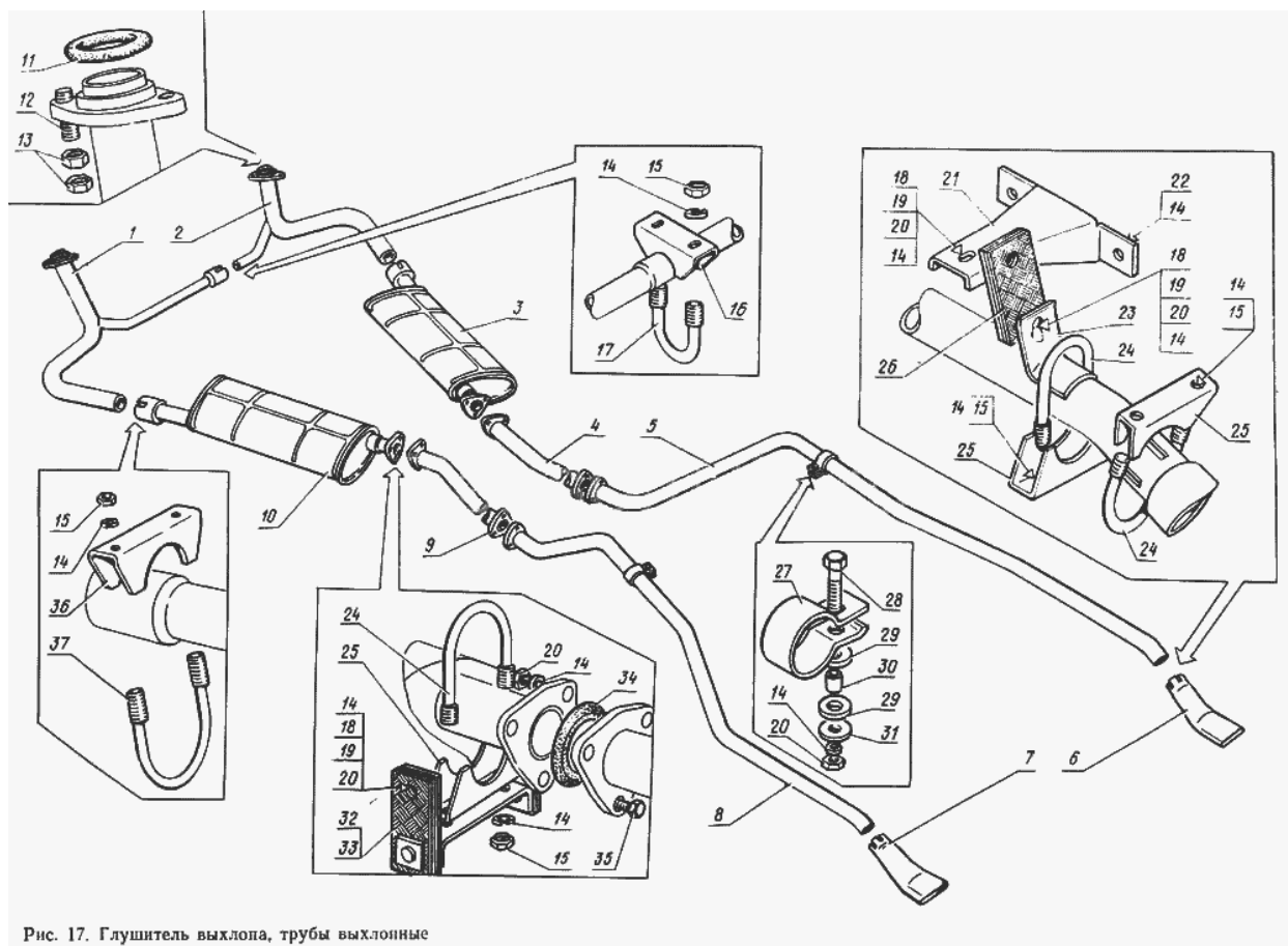
Рис. 17. Глушитель выхлопа, трубы выхлопные
