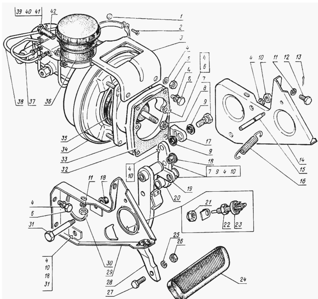
Рис. 48. Педаль и привод механизма управления тормозами, главный цилиндр тормозов, вакуумный усилитель тормозов
