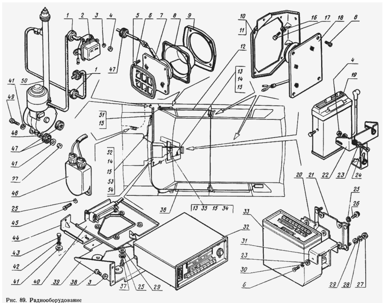
Рис. 89. Радиооборудование
