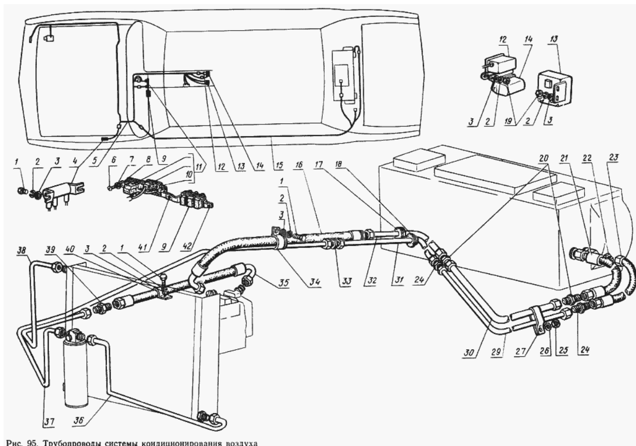
Рис. 95. Трубопроводы системы кондиционирования воздуха
