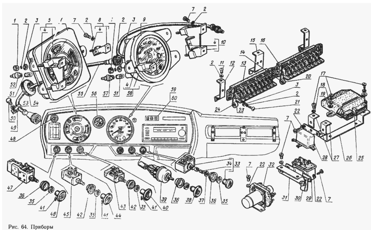
Рис. 64. Приборы
