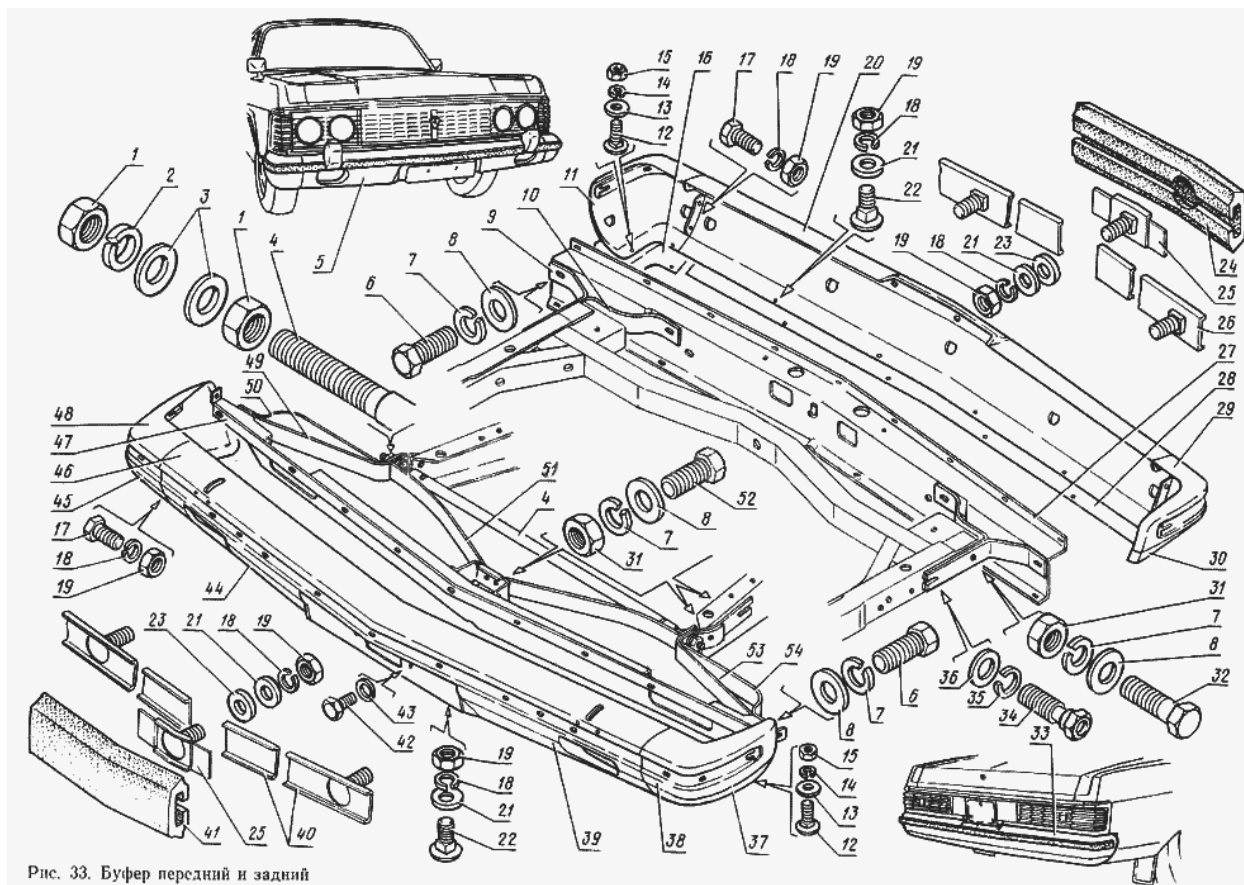
Рис. 33. Буфер передний и задний
