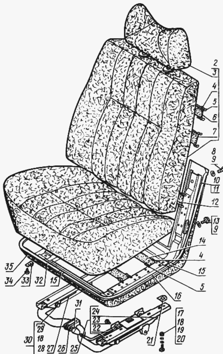
Рис. 85. Сиденье водителя и механизм регулирования положения сиденья водителя
