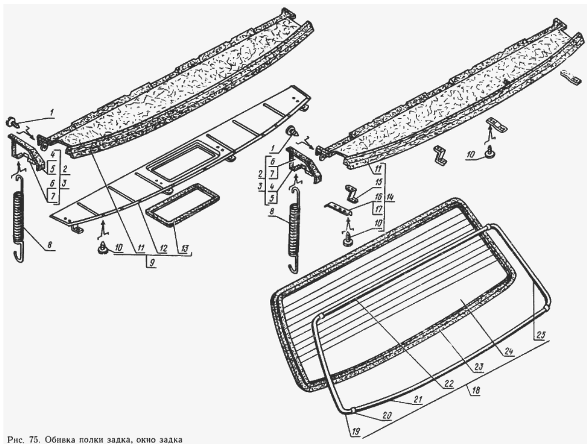
Рис. 75. Обивка полки задка, окно задка
