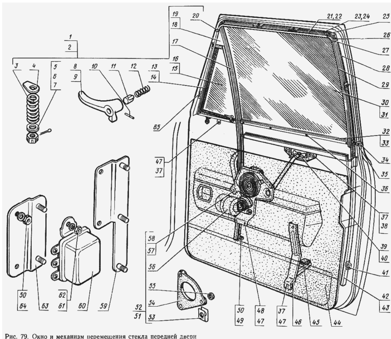
Рис. 79. Окно и механизм перемещения стекла передней двери
