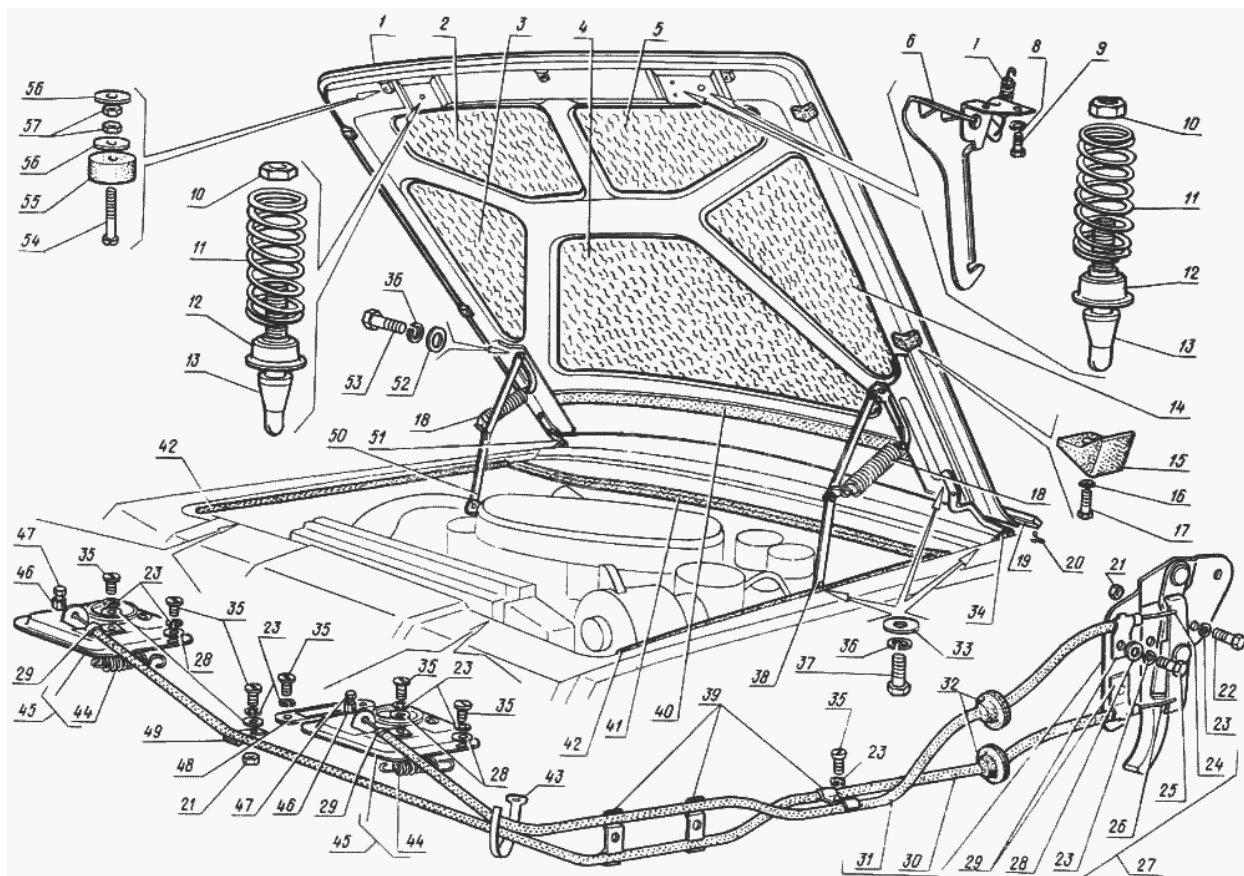
Рис. 98. Капот, замок и привод замка капота, навеска и упор капота
