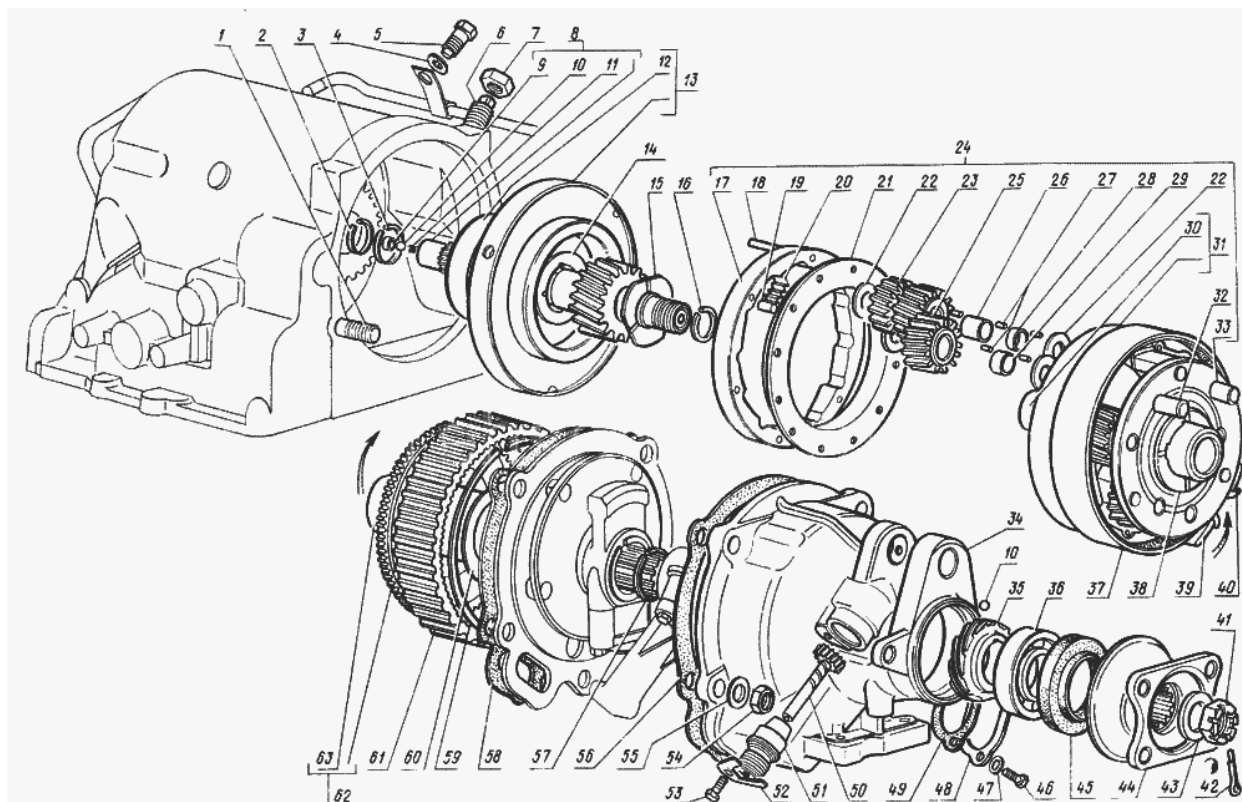
Рис. 25. Механизм планетарный коробки передач
