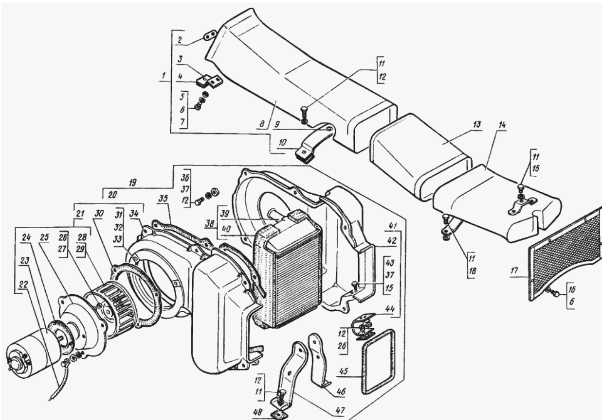
Рис. 91. Распределитель воздухообогрева, крепление заднего отопителя, отопитель кузова задний
