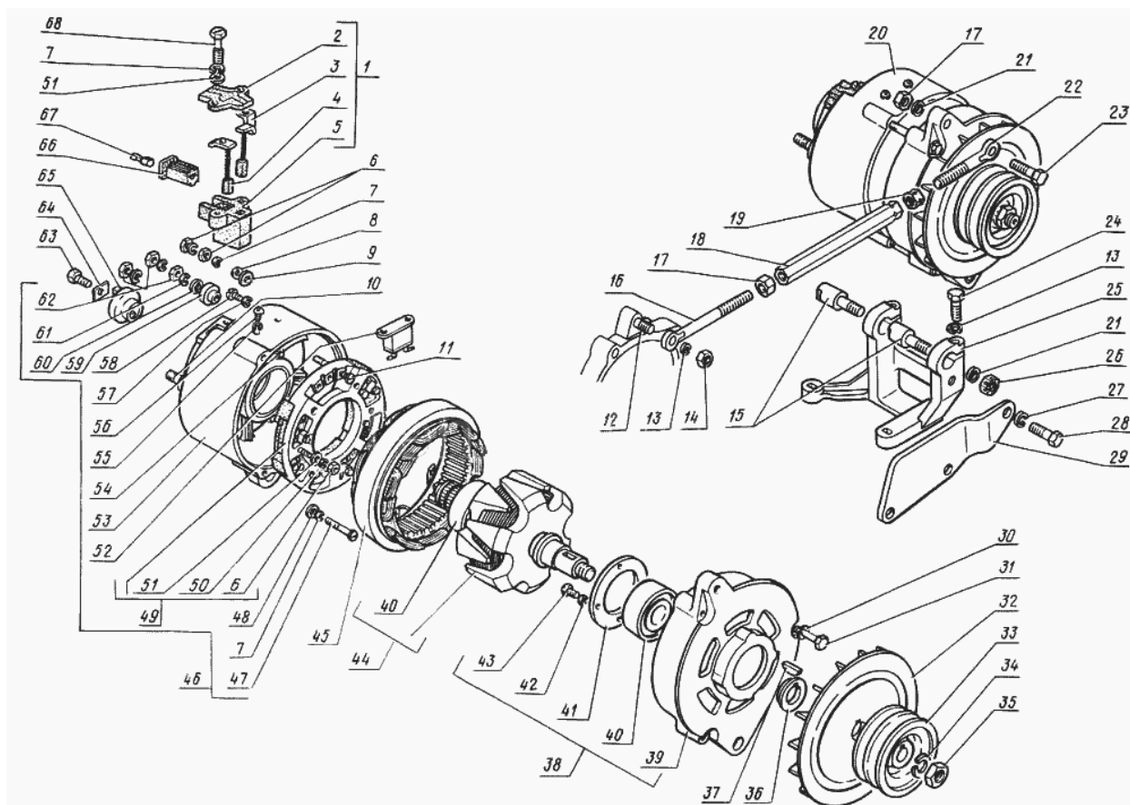
Рис. 52. Генератор
