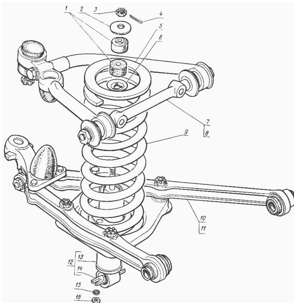
Рис. 35. Пружины, рычаги передней подвески в сборе и крепление передних амортизаторов
