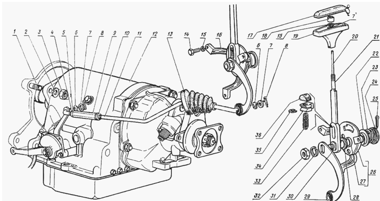
Рис. 21. Коробка передач автоматическая и привод управления ручным золотником коробки передач
