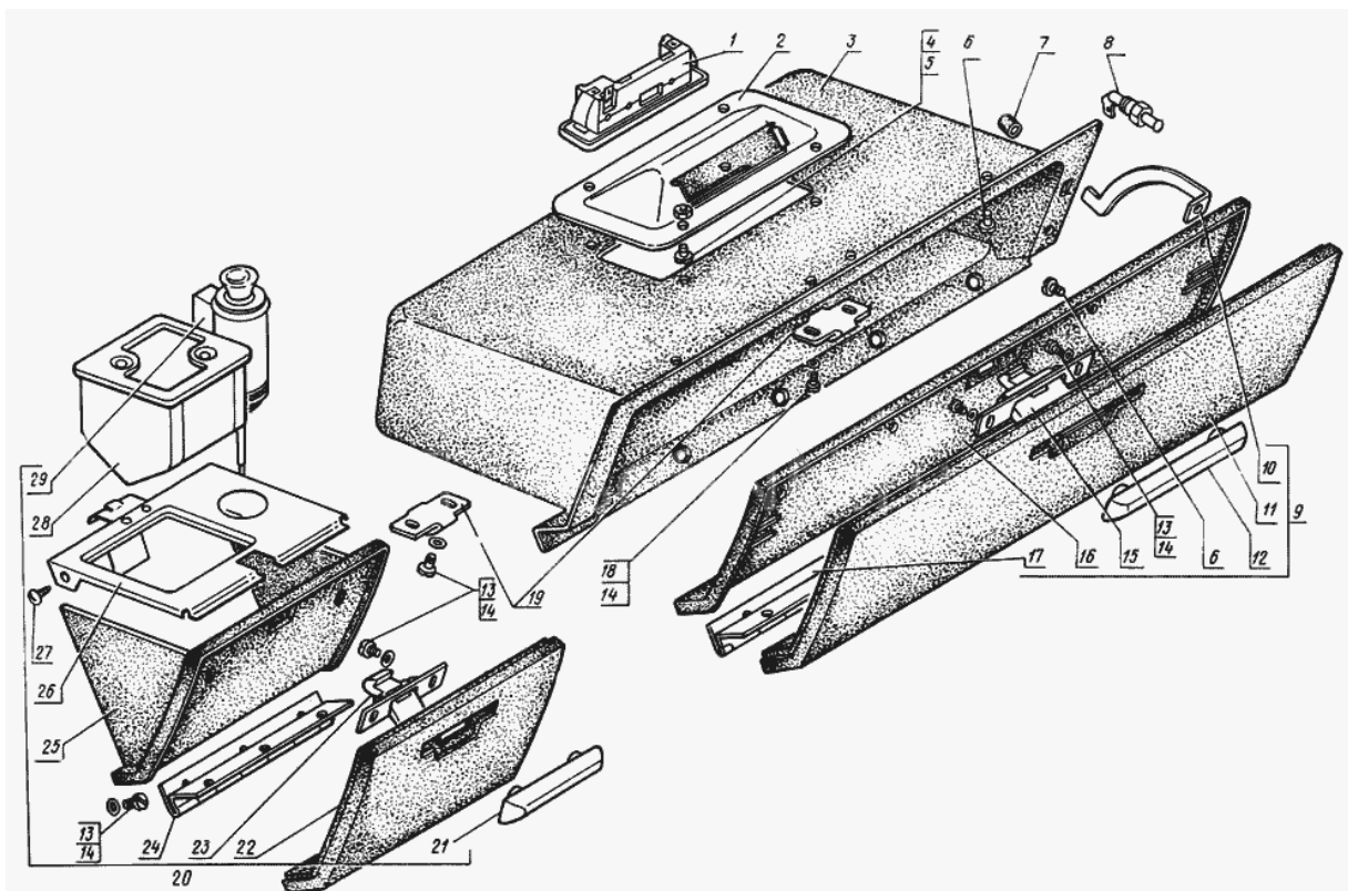
Рис. 69. Ящик вещевой и пепельница передняя
