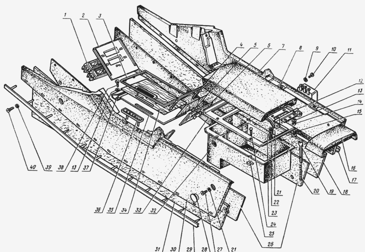
Рис. 71. Консоль панели приборов
