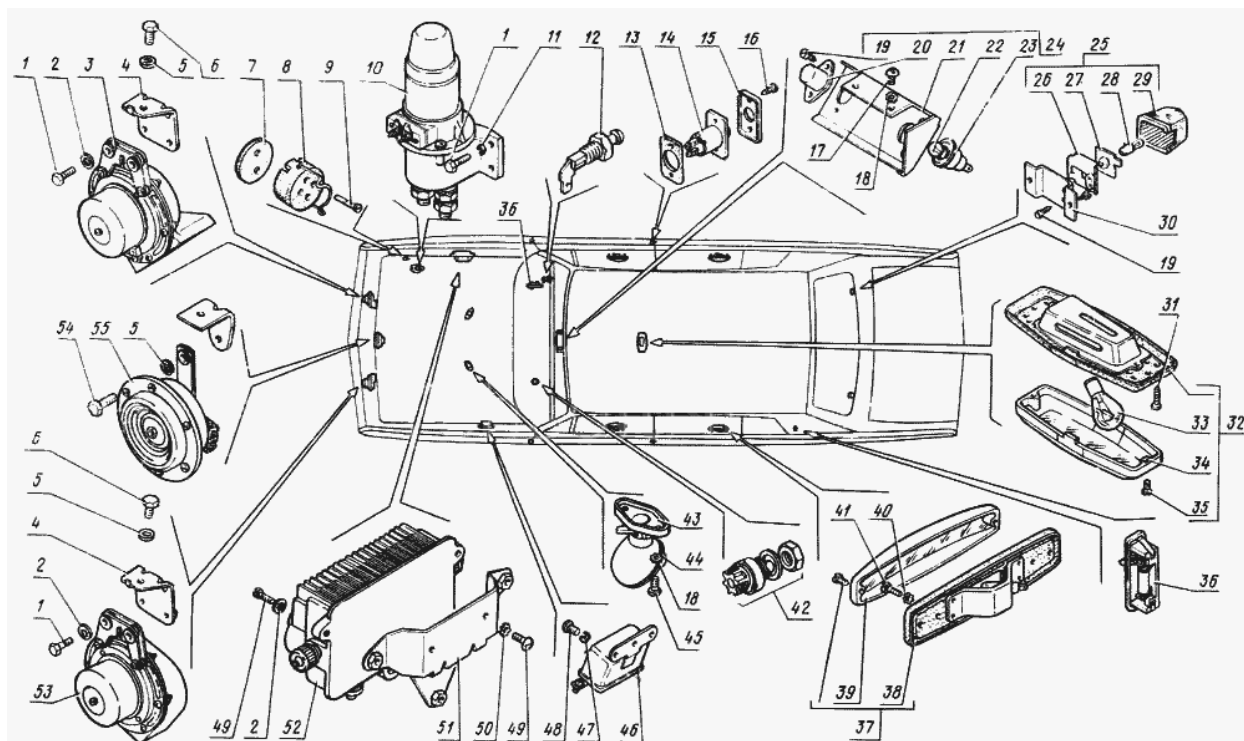
Рис. 59. Внутреннее освещение, сигналы звуковые, коммутатор транзисторный, выключатель массы
