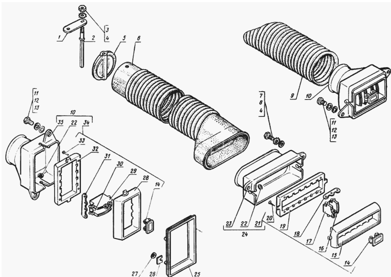
Рис. 92. Вентиляция кузова, обогрев боковых стекол
