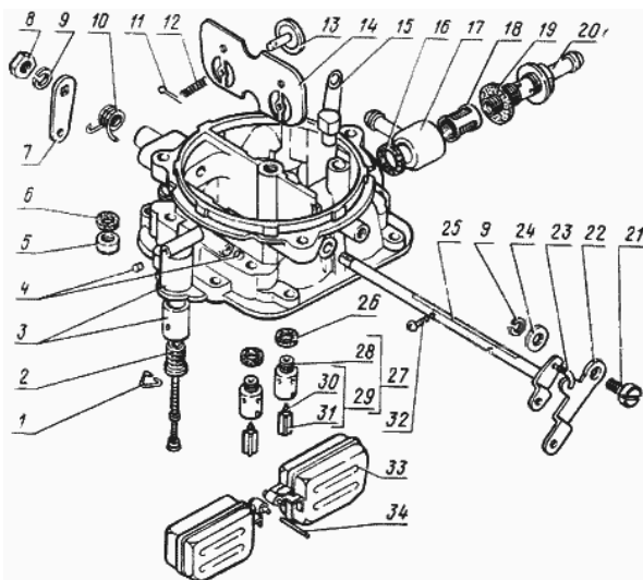
Рис. 12. Карбюратор
