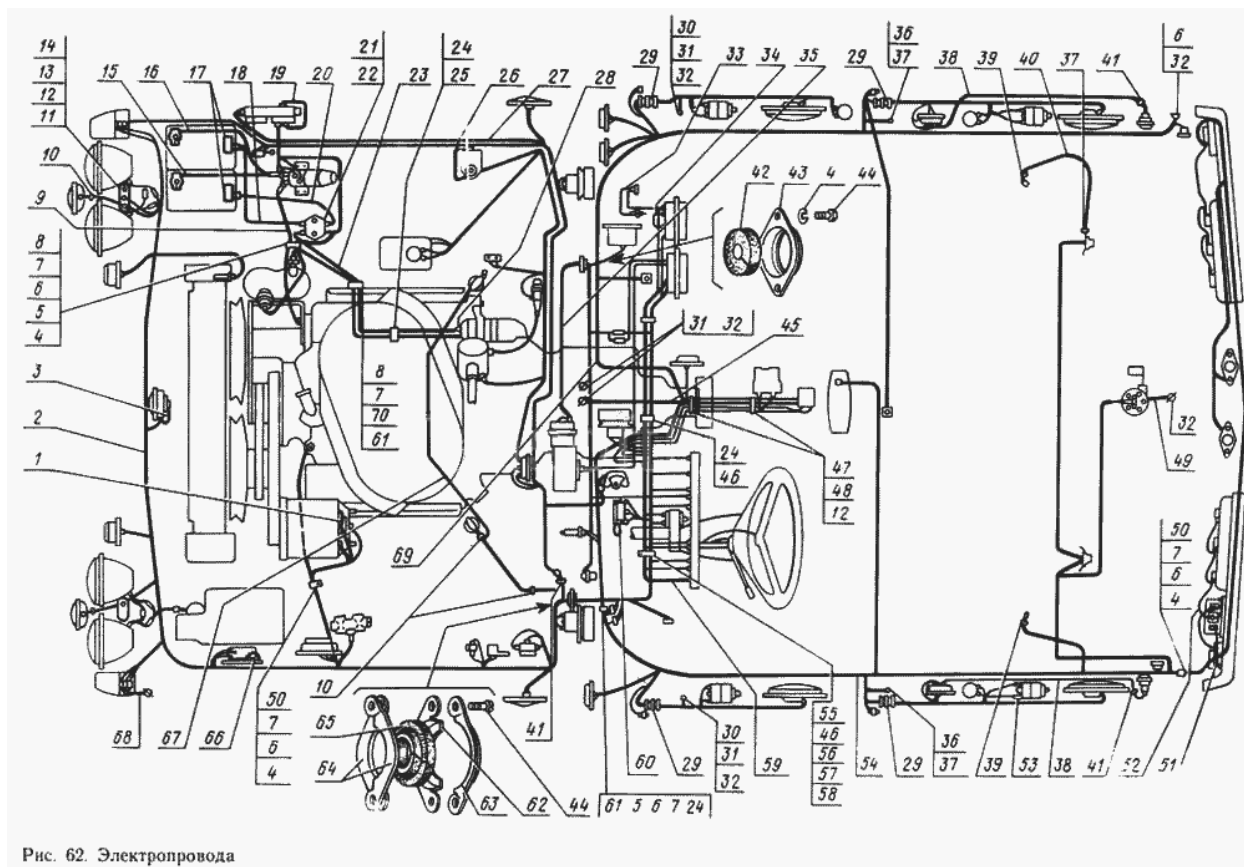
Рис. 62. Электропровода
